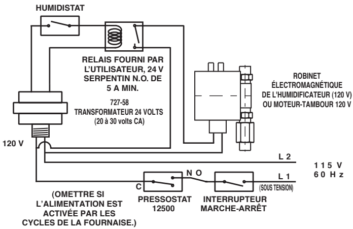
SCHÉMA 3 CÂBLAGE DE L'HUMIDIFICATEUR DE PUISSANCE 1137 (120 VOLTS)
