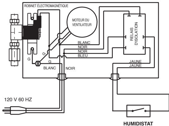
SCHÉMA 4 HUMIDIFICATEUR À INJECTION DE VAPEUR ELITE AVEC CABLAGE DE 230 V
