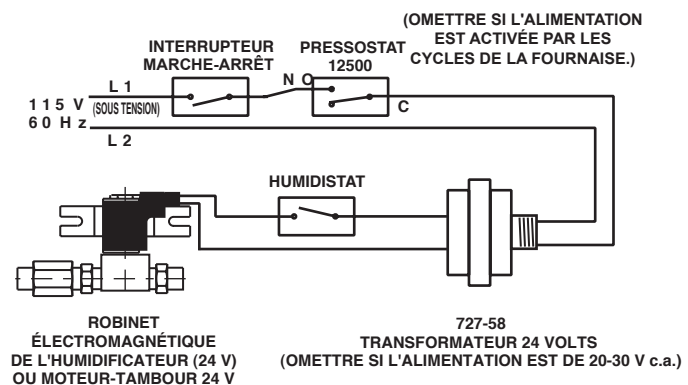
SCHÉMA 1 CÂBLAGE DE L'HUMIDIFICATEUR EN DÉRIVATION (24 VOLTS)
