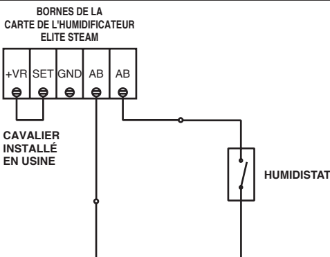
SCHÉMA 5 HUMIDIFICATEUR À INJECTION DE VAPEUR ELITE AVEC CÂBLAGE DE 230 V
