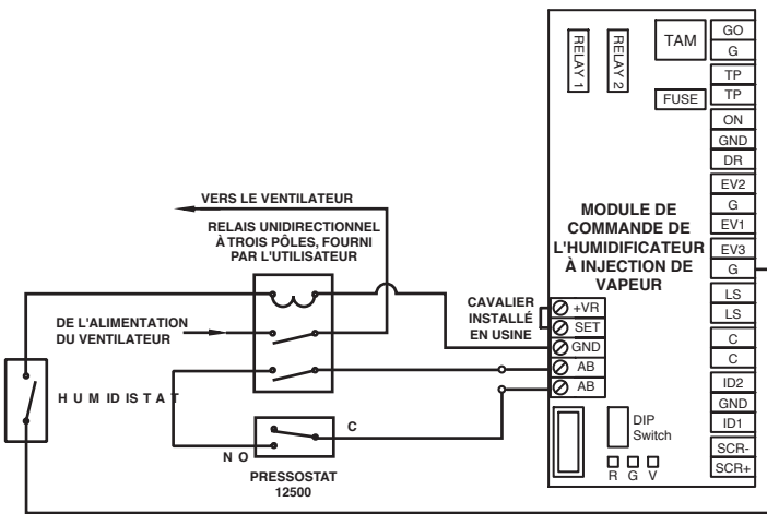
SCHÉMA 5 HUMIDIFICATEUR À INJECTION DE VAPEUR ELITE AVEC CÂBLAGE DE 230 V
