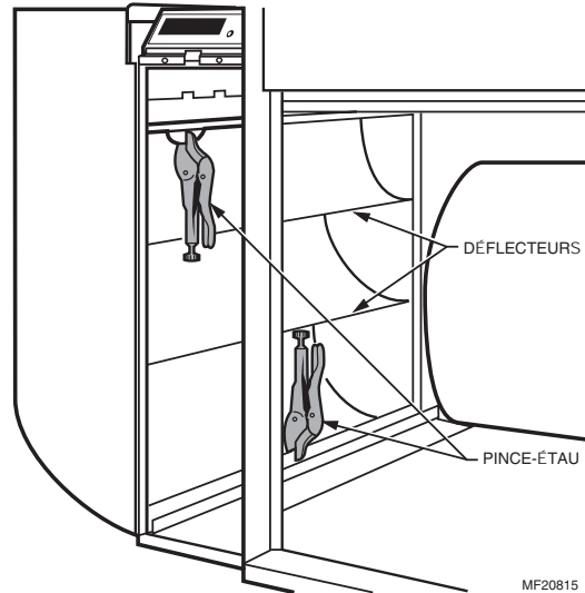
Fig. 6. Fixer la gaine d'air au filtre à air. Noter la position des déflecteurs. La pince-étau sert à tenir ensemble l'appareil et la gaine d'air pendant l'installation.
