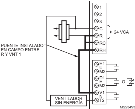
Conexión típica de ventilación sin energía.
